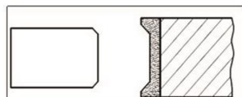
Trapezia edge wheel (FA) Glass 3MM-19MM
