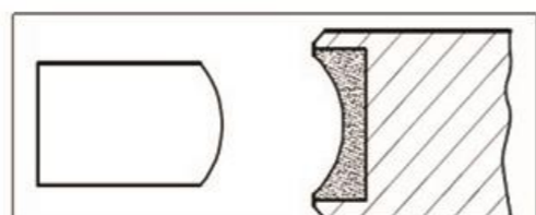
Pencil edge wheel (PE) Glass 3MM-19MM
